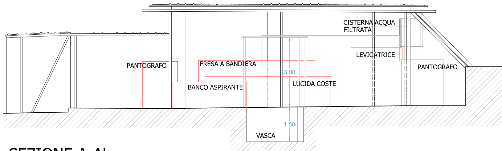
SEZIONE A-A'
