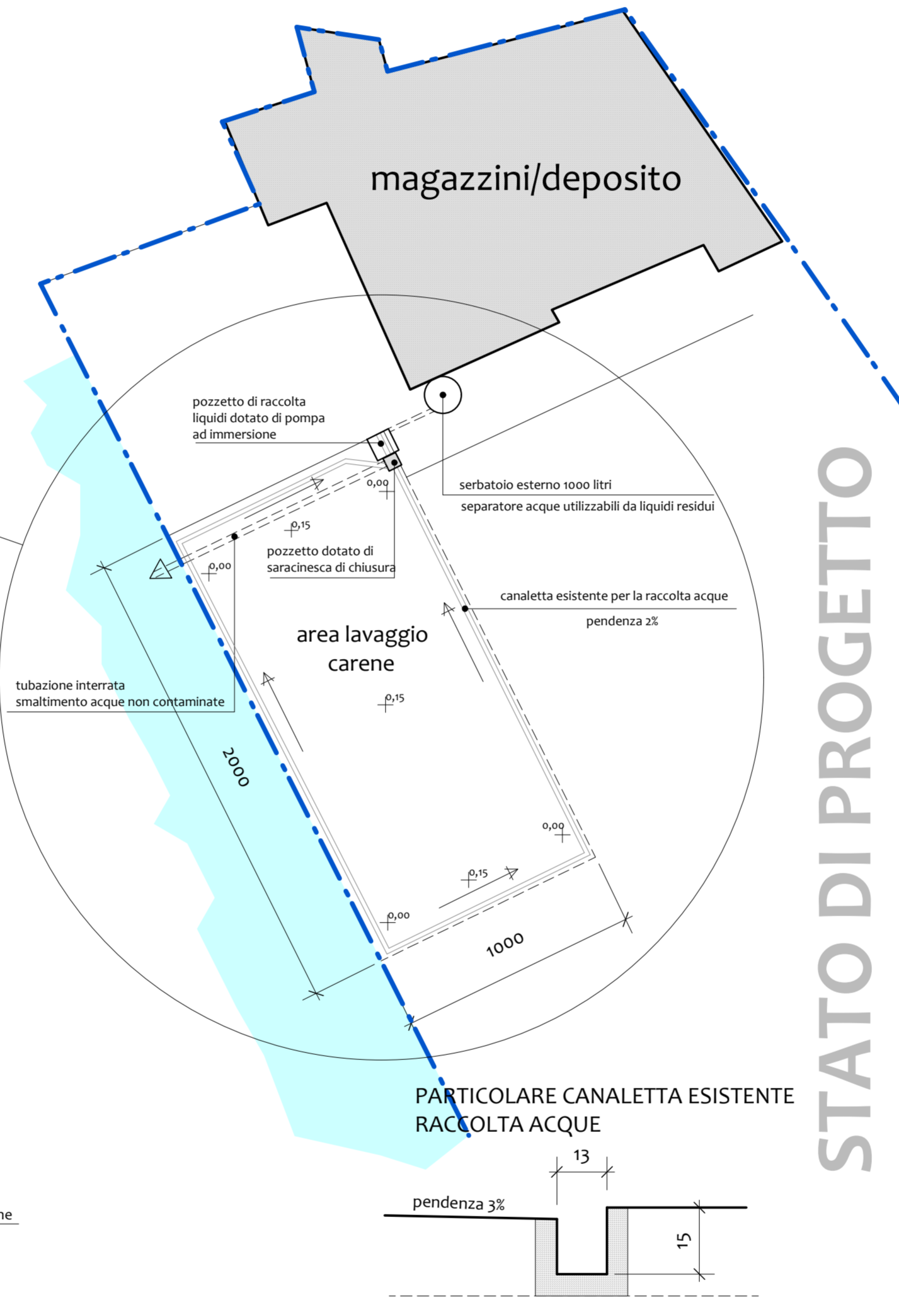
PARTICOLARE SISTEMA DI SMALTIMENTO ACQUE REFLUE scala 1:200
