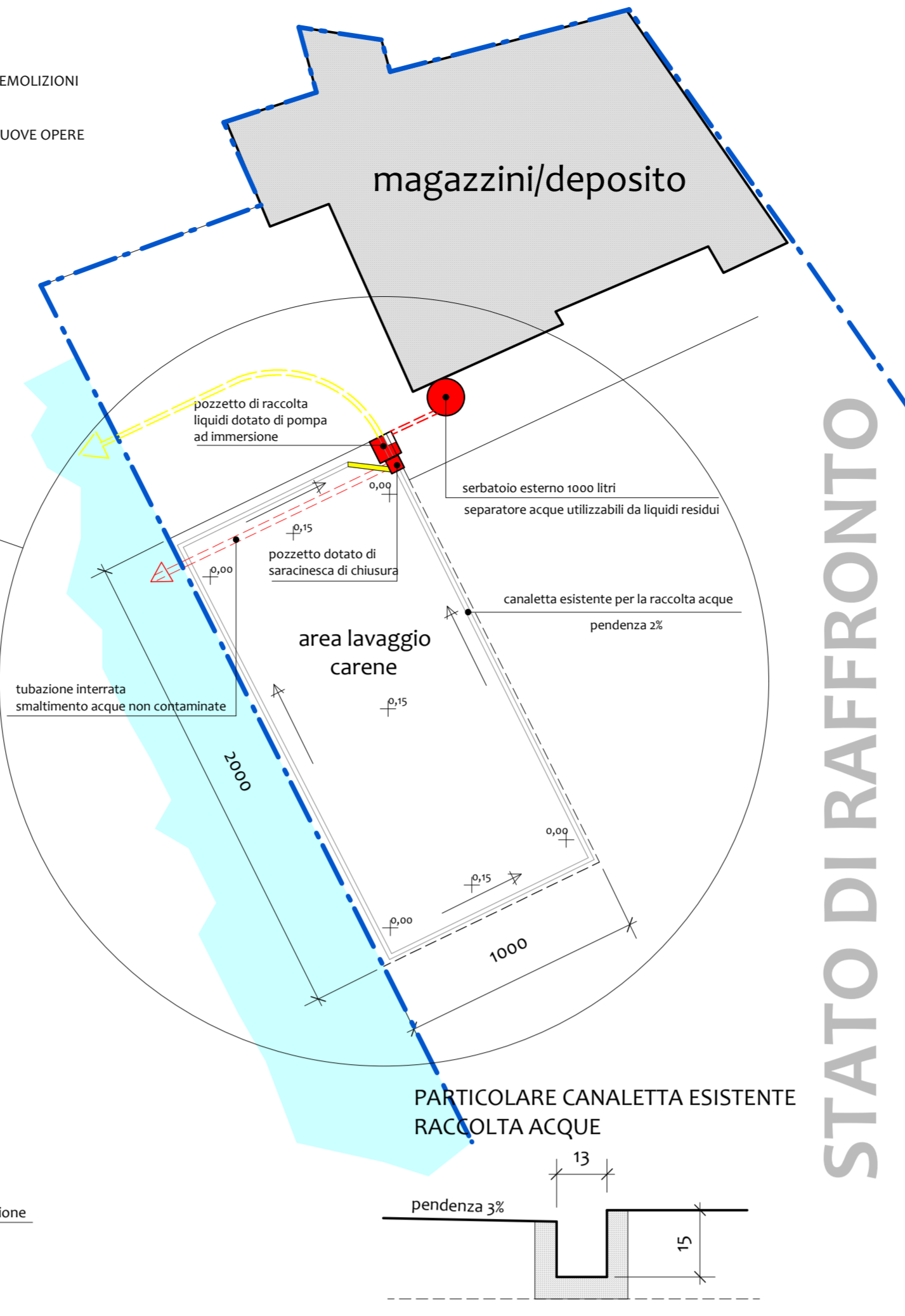
PARTICOLARE SISTEMA DI SMALTIMENTO ACQUE REFLUE scala 1:200
