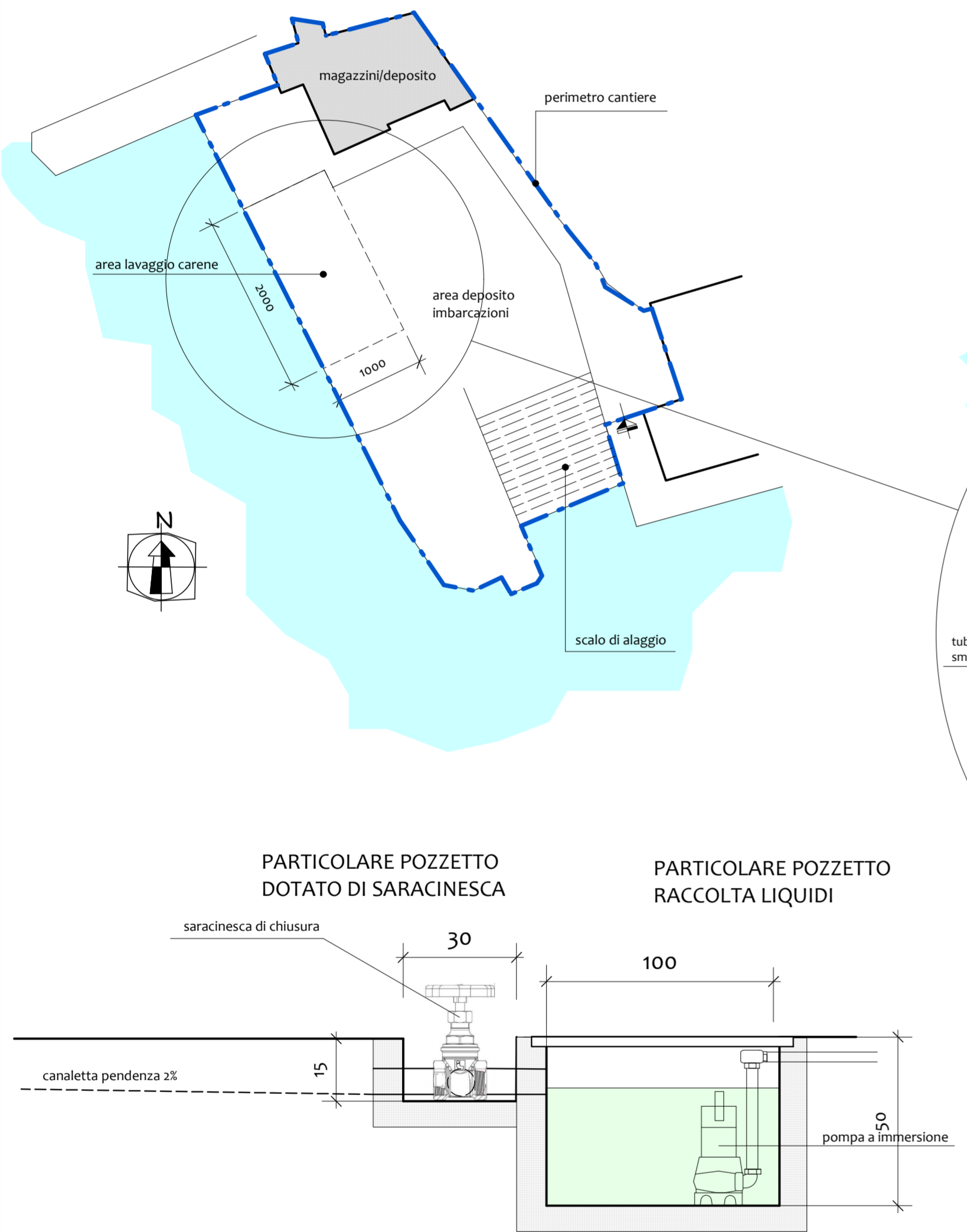
PLANIMETRIA AREA CANTIERE NAVELE DI CAMOGLI s.r.l. scala 1:500
