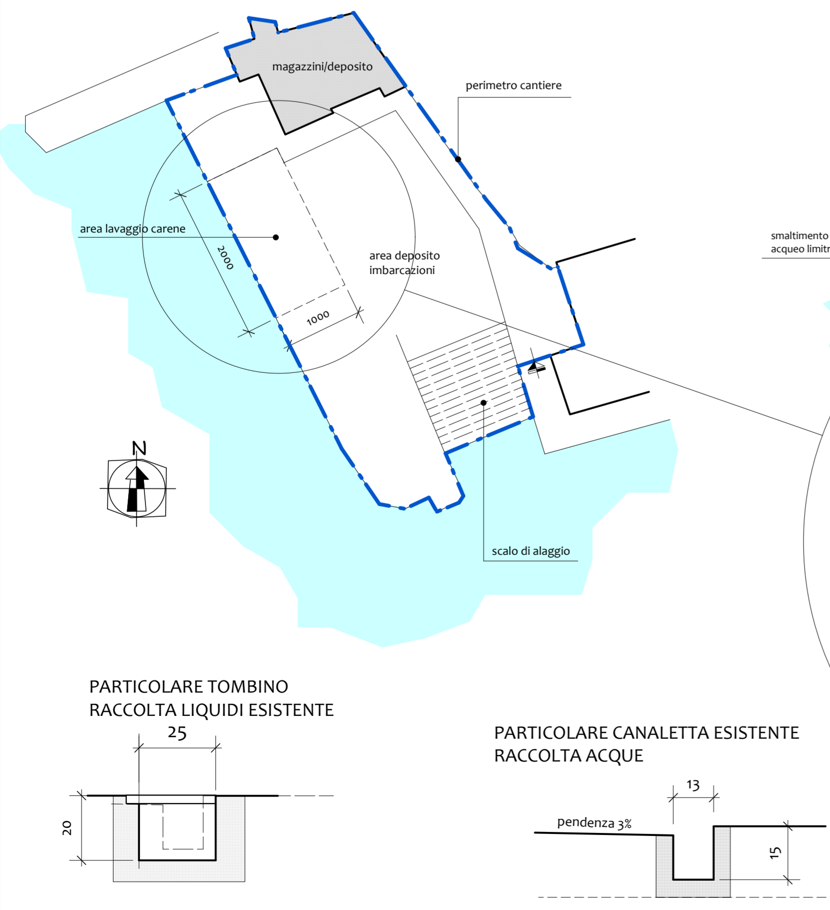
PLANIMETRIA AREA CANTIERE NAVELE DI CAMOGLI s.r.l. STATO ATTUALE - scala 1:500
